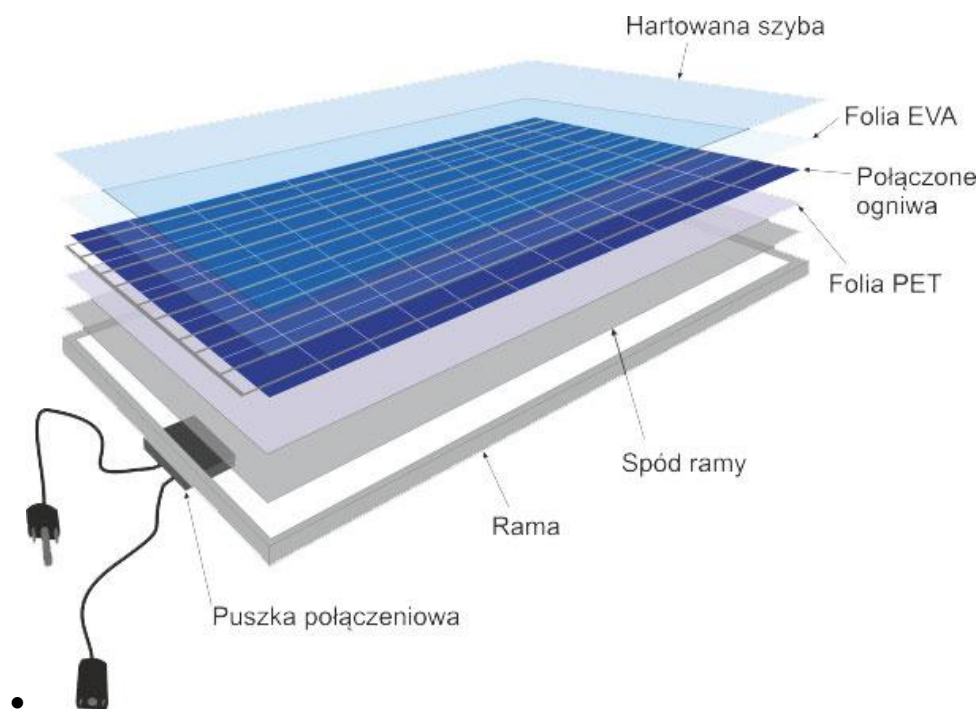
Rysunek 9 Powyższe foto przedstawia przekrój modułu PV polikrystalicznego i monokrystalicznego
