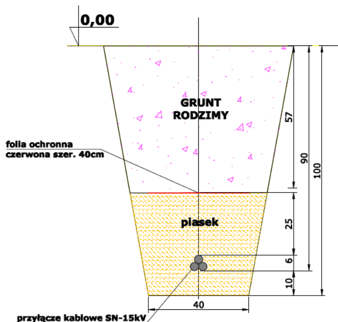
Rysunek 13 Sposób ułożenie przylącza w gruncie
