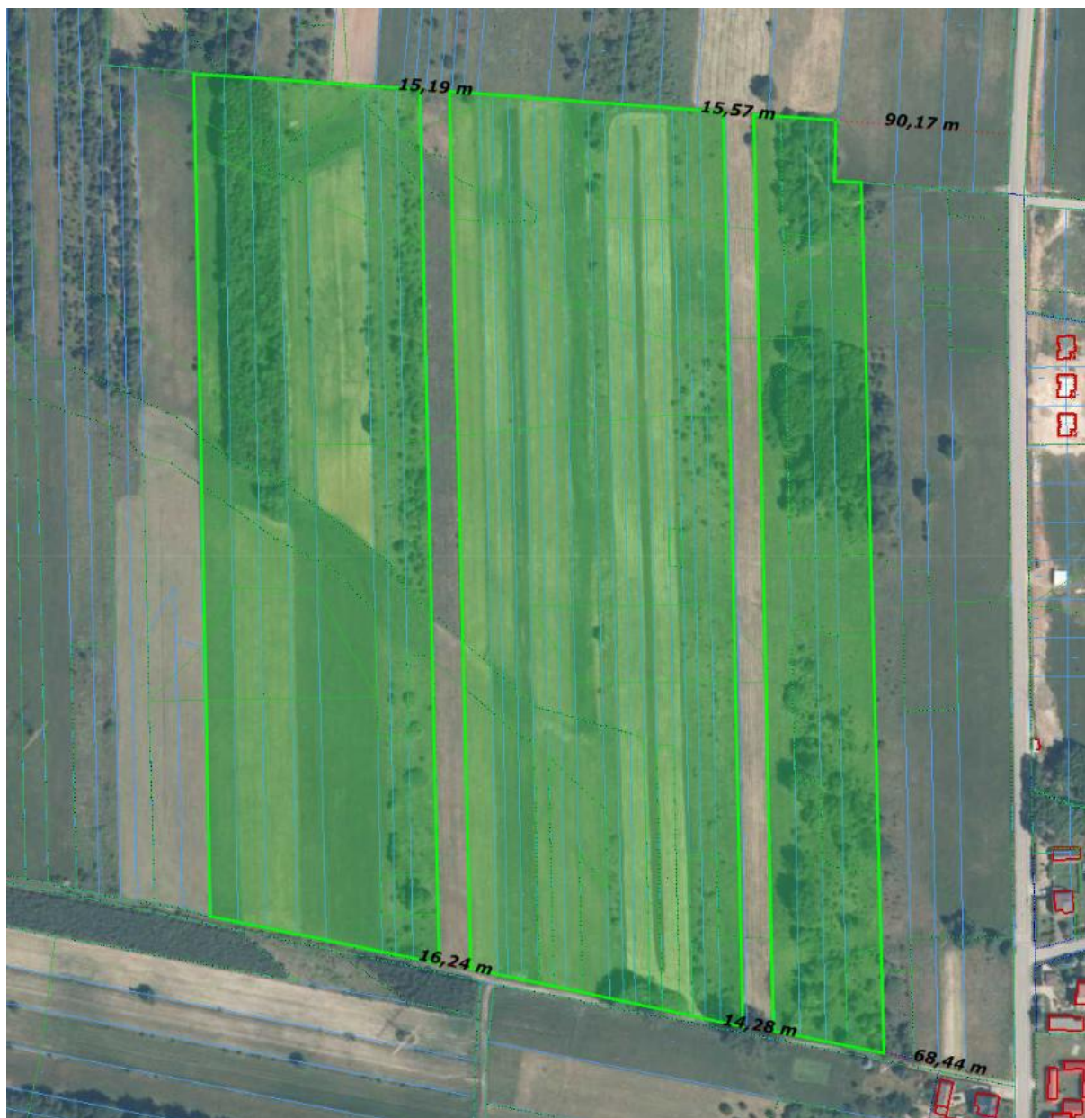
Mapa 4 Podział terenu inwestycji na sektory zabudowy panelami fotowoltaicznymi oraz pasy otwarte umożliwiające migrację zwierząt.
