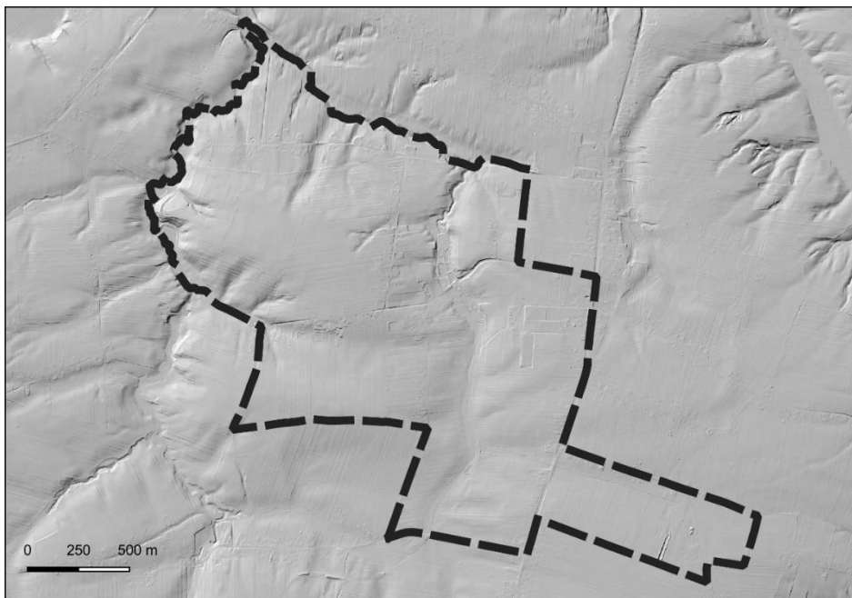
Rys. 3 Ukształtowanie terenu opracowania.
