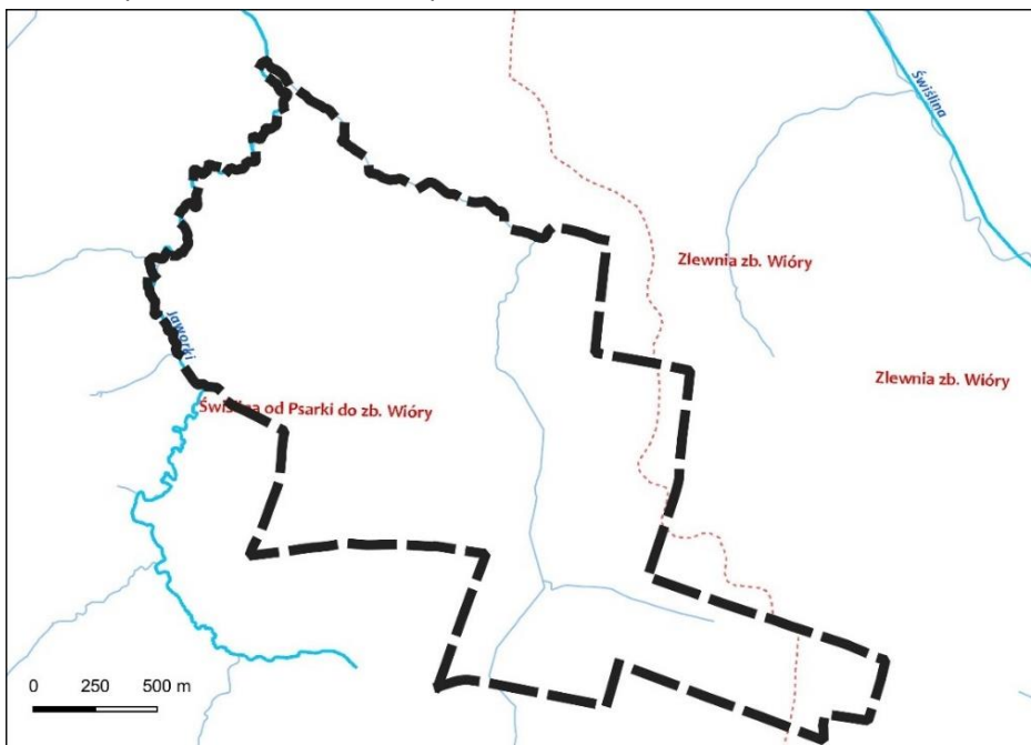
Rys. 4 Zlewnie poziomu 5 na terenie opracowania.
