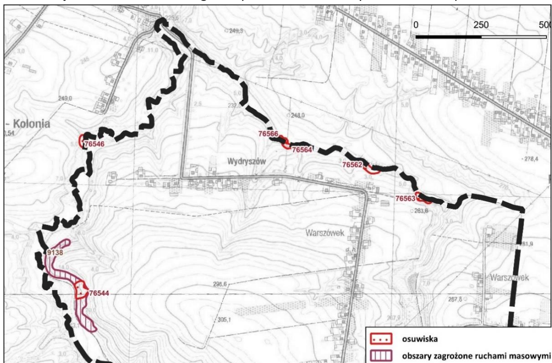
Rys. 11 Lokalizacja osuwisk i terenów zagrożonych ruchami masowymi na terenie opracowania.
