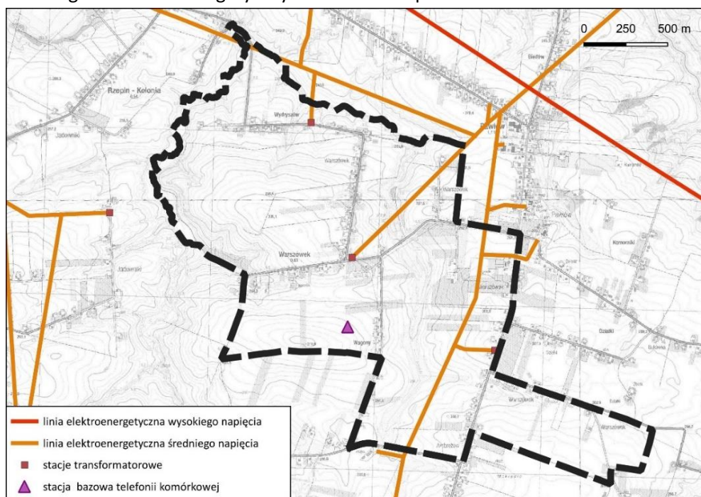
Rys. 9 Przebieg linii elektroenergetycznych na terenie opracowania.
